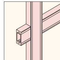
見付け 20mmタイプ
