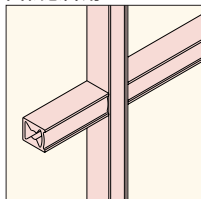
見付け 7mmタイプ
